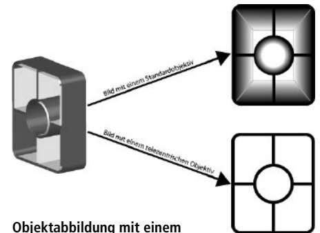
Objektabbildung mit einem telezentrischen Objektiv
